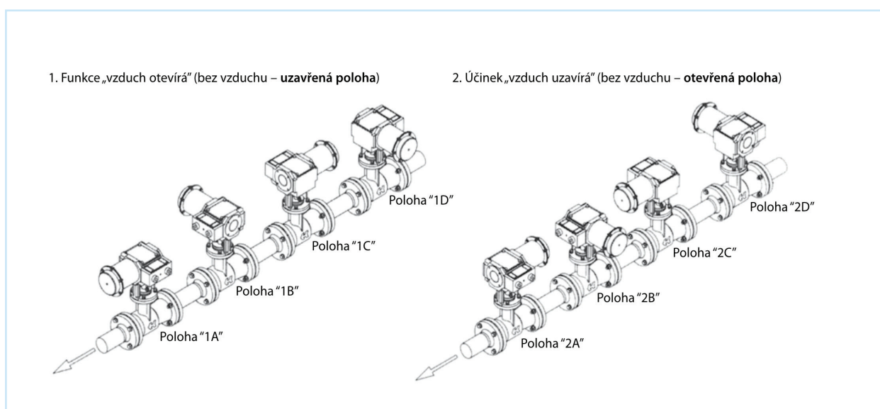
OBR. 5 VARIANTY MOŽNÝCH NASTAVENÍ SERVOPOHONU TYP RP99 VŮČI OSE VENTILU
