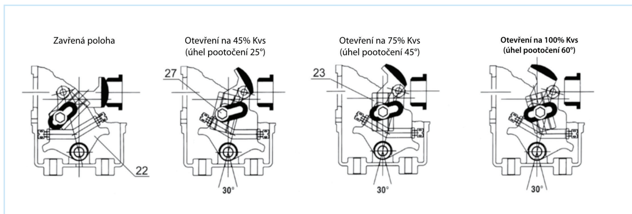
OBR. 4B - VARIANTY NASTAVENÍ ČEPU LOŽISKA(27) NA PÁCE(22) V ZÁVISLOSTI NA ÚHLU POOTOČENÍ OJNICE(23) (HŘÍDELE VENTILU - HODNOTY KVS)
