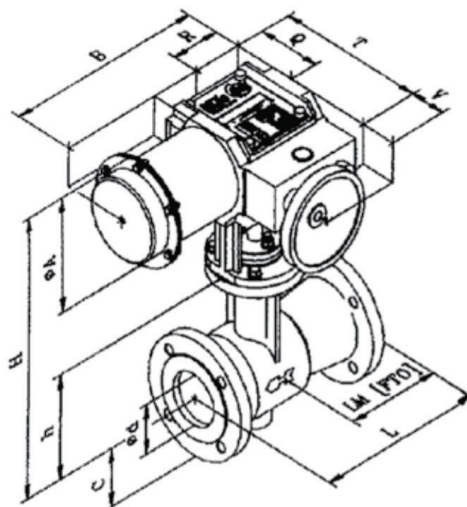
Přírubový ventil Pohon RP99-1
