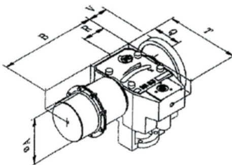
Servopohon RP99-2 Servopohon RP99-3
