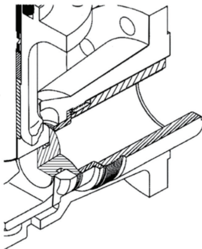
Kuželka, sedlo a prodloužená šroubová zátka z vytvrzeného materiálu - antierozní provedení
