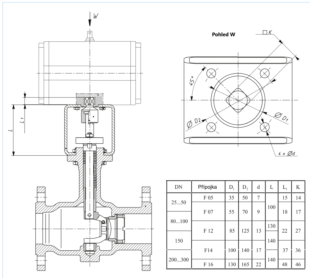
OBR. 9 - VÝKRES PŘIPOJOVACÍCH ROZMĚRŮ
