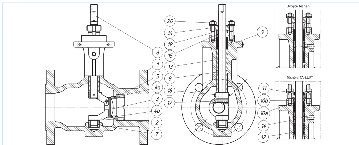
OBR. 1 - VENTIL TYPU VA3033
