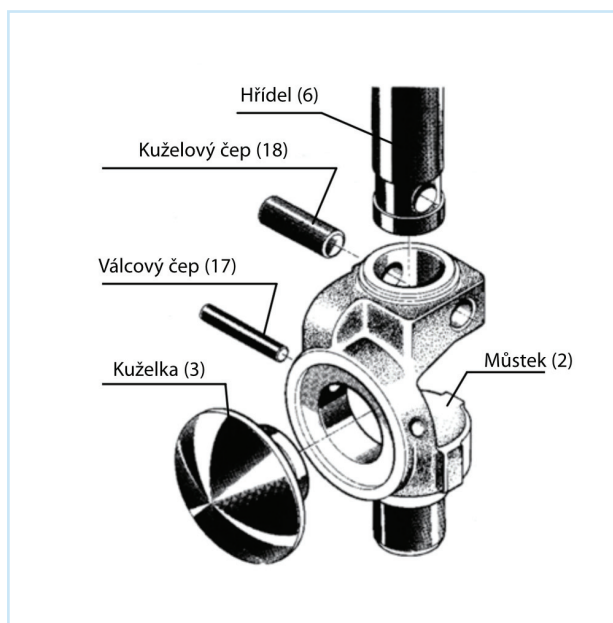
FIG. 4A - POHON TYPU RP99
