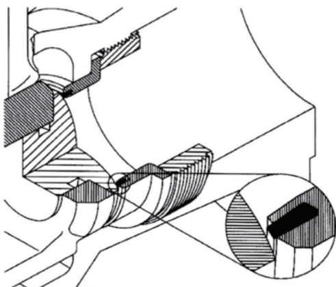
Těsnění PTFE „měkké“ - zaručuje bublinkovou těsnost (VI tř.)
