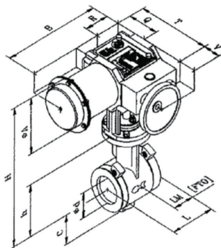
Ventil bez přírub - Sandwich Pohon RP99-1
