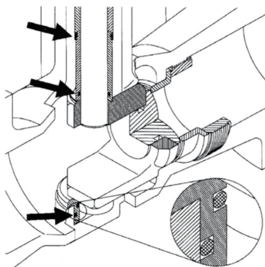
Těsnění vodicích pouzder pro chlor a krystalizující média
